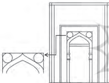
تصویر ۲۰. ساختار محراب داخلی مسجد کرمانی تربت جام، ماخذ: همان. تصویر ۲۱. قرار گرفتن فرم‌گرد در لچکی محراب داخلی مسجد کرمانی تربت جام، ماخذ: همان.
