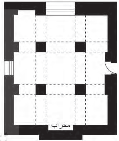
نقشه ۳. پلان طبقه اول مسجد کوچه میر نطنز و موقعیت قرارگیری محراب در آن (برداشت و ترسیم نگارندگان)
