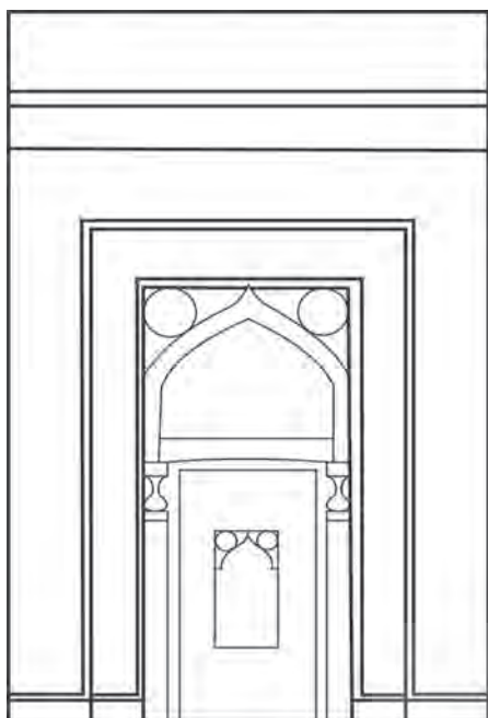
تصویر ۱. ساختار محراب امامزاده ربیع‌خاتون اشترجان (نگارندگان)
