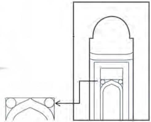
تصویر ۲۶. ساختار محراب طبقه دوم مسجد کوچه میر نطنز، ماخذ: همان. تصویر ۲۷. قرار گرفتن فرم گرد در لچکی محراب طبقه دوم مسجد کوچه میر نطنز، ماخذ: همان.
