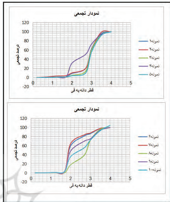
نگاره ۷: نمودار تجمعی نمونه‌ها
