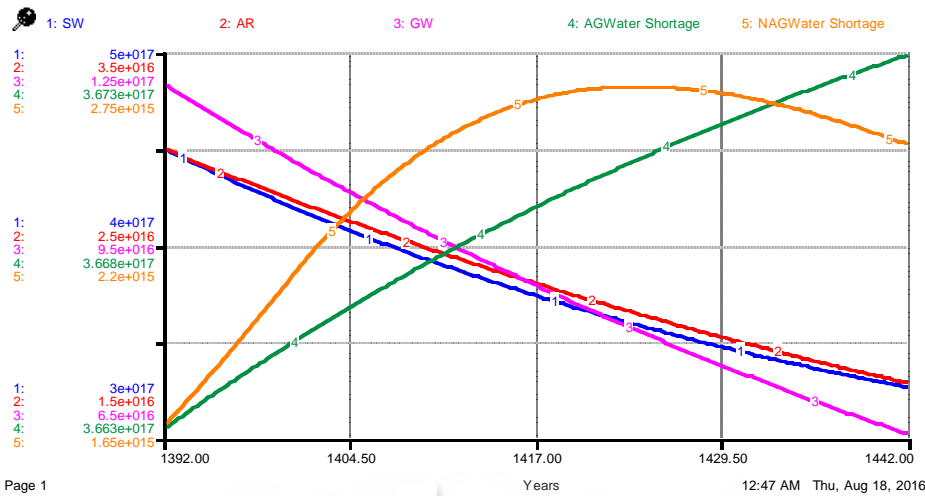
شکل ۳- روند تخلیه آب‌های سطحی (SW)، زیرزمینی (GW) و ذخیره‌شده (AR) و روند کمبود آب در بخش‌های کشاورزی (AGWaterShortage) و غیر کشاورزی (NAGWaterShortage) (واحد متغیرها میلی‌متر مکعب)
