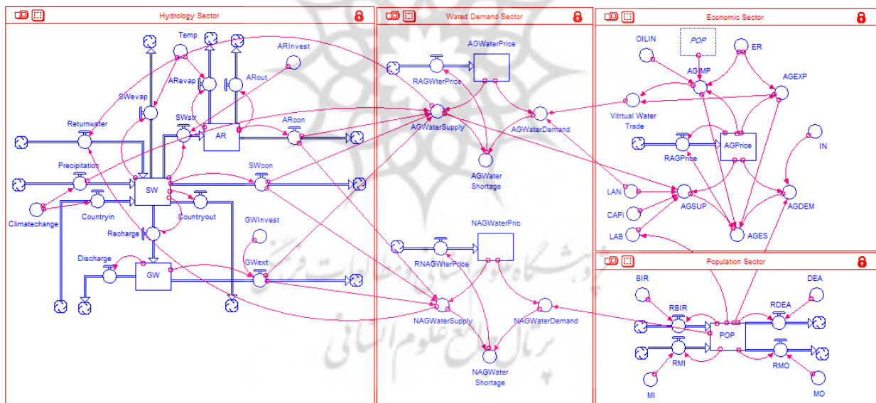
شکل ۲- مدل ذخیره-جریان برای کل بخشهای هیدرولوژی، تقاضا برای آب، اقتصادی و اجتماعی
