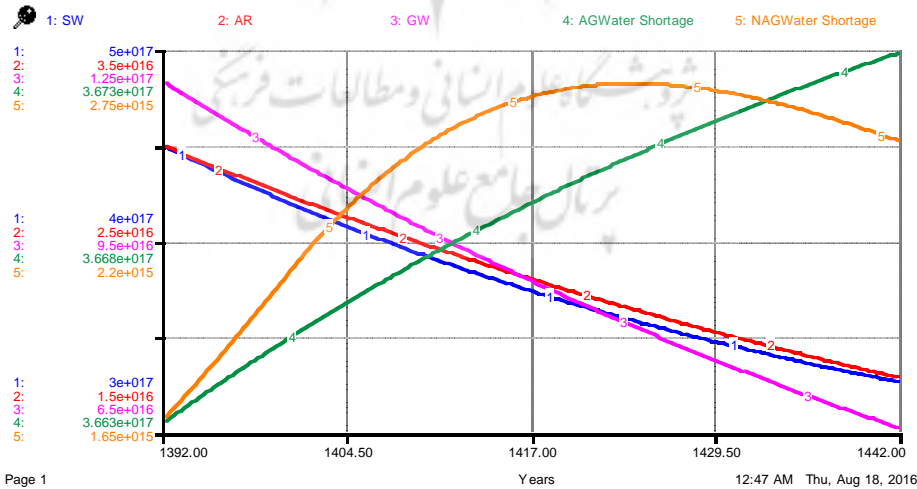
شکل ۱- روند تخلیه آب‌های سطحی (SW)، زیرزمینی (GW) و ذخیره‌شده (AR) و روند کمبود آب در بخش‌های کشاورزی (AGWaterShortage) و غیر کشاورزی (NAGWaterShortage) - (واحد متغیرها میلی‌متر مکعب) Figure 1-The depletion trend of surface water (SW), groundwater aquifers (GW) and reservoir (AR) and non-agricultural water shortages (NAGWaterShortage)- (mm 3 )
