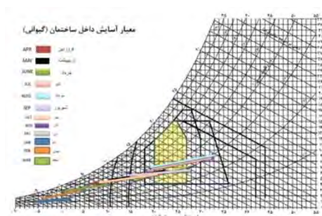
نمودار ۵: نمودار معیار زیست اقلیم گیوانی، منبع: نگارندگان
