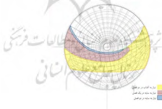
تصویر ۳: انتقال مواقع نیاز به سایه و آفتاب از تقویم نیاز اقلیمی بر نقشه مسیر خورشید و همپوشانی آن با نقاله سایه یاب، منبع: نگارندگان
