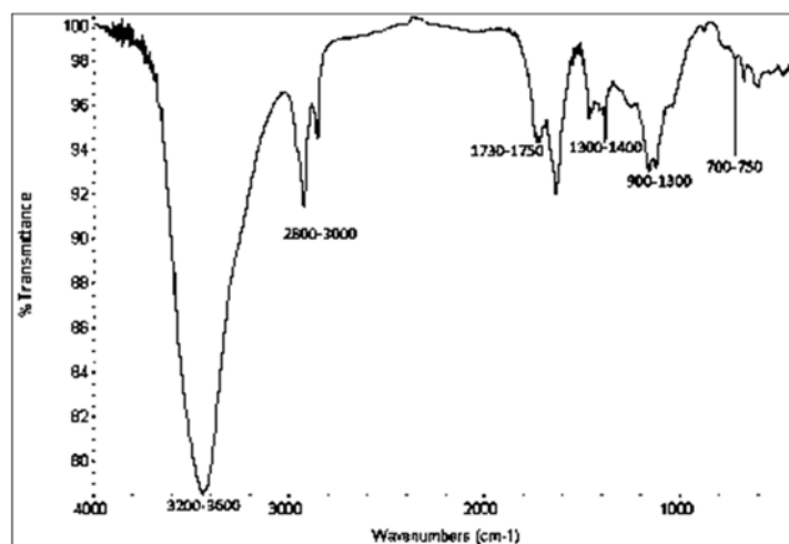
شکل ۶: طیف FTIR از ماده‌ی چسباننده‌ی ورق طلا در طلاچسبان کتیبه‌ی سنگی کلیسای وانک
