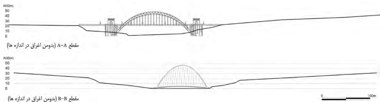
تصویر ۲: با مقایسه فرمی پل میلیوم با پل تاین این حقیقت آشکار می‌شود که پل جدیدتر از نظر شکل و ارتفاع، دنباله‌رو پل قبلی است اما با زبانی مدرن، مأخذ: stnatlusnoC esU dnaL, ۳۰۰۲: ۳۴.
