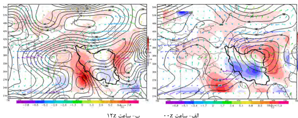
شکل ۶: نقشه همگرایی و واگرایی شار رطوبت ( 10^{-5} \text{ g.kg}^{-1} . \text{s}^{-1} ) سطح ۸۵۰ ه.ب، ارتفاع ژئوپتانسیل (m) و وزش دمایی ( ^{\circ}\text{C} ) سطح ۱۰۰۰ ه.پ، ۶ ژانویه ۲۰۰۹
