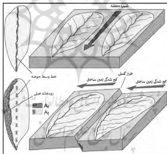
شکل ۴: بلوک دیاگرام نشانگر نحوه محاسبه فاکتور عدم تقارن حوضه زهکشی (AF) (Mahmood and Gloaguen, 2012).
