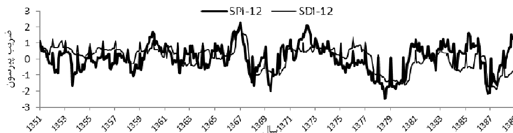
شکل ۸: نمودار SPI و SDI ۱۲ ماهه برای حوضه صوفی چای
