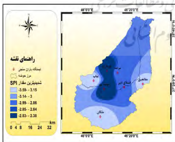
شکل ۶: گستره شدیدترین خشکسالی‌ها در مقیاس زمانی ۱۲ ماهه
