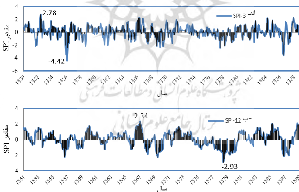
شکل ۲: نمودار وضعیت ترسالی‌ها و خشکسالی‌های هواشناسی ایستگاه مراغه در بازه‌های زمانی الف) ۳ ماهه و ب) ۱۲ ماهه
