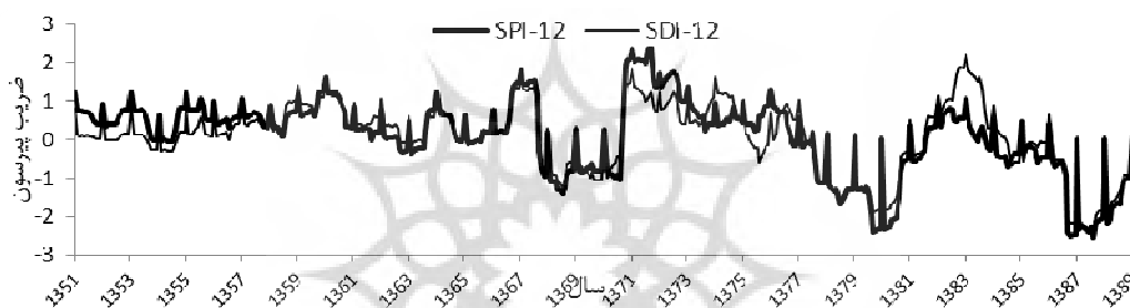
شکل ۹: نمودار SPI و SDI ۱۲ ماهه برای حوضه مردق چای
