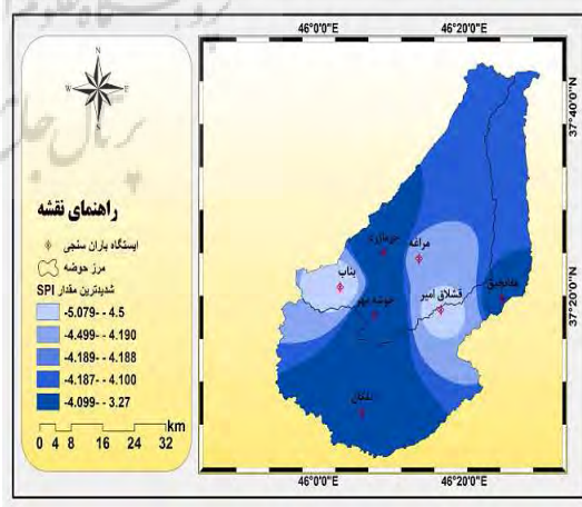
شکل ۵: گستره شدیدترین خشکسالی‌ها در مقیاس زمانی ۳ ماهه
