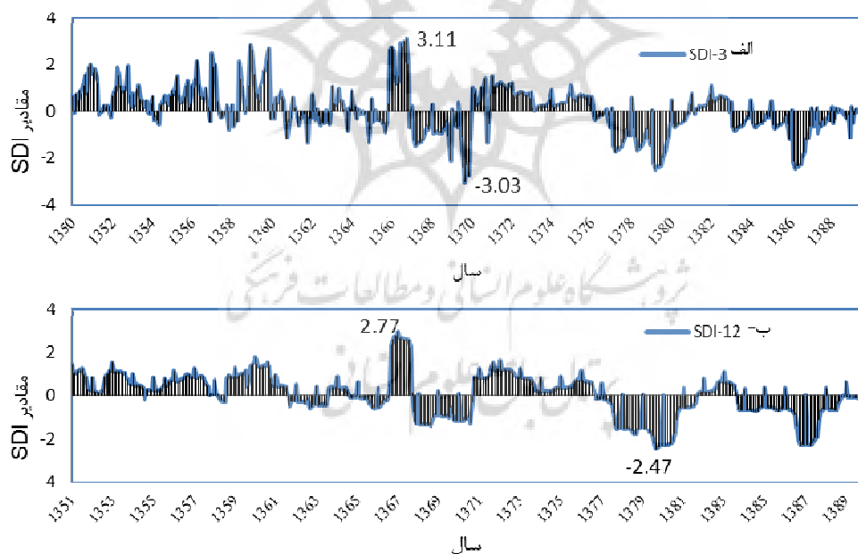
شکل ۷: نمودار وضعیت ترسالی‌ها و خشکسالی‌های هیدرولوژیکی ایستگاه مراغه در بازه‌های زمانی الف) ۳ ماهه و ب) ۱۲ ماهه
