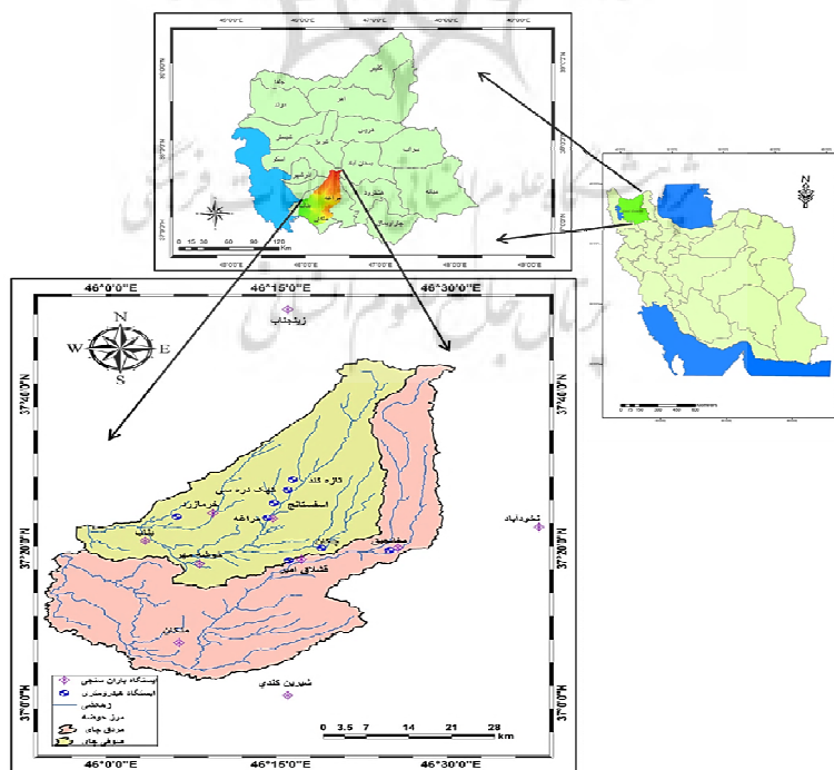
شکل ۱: نقشه موقعیت منطقه مورد مطالعه به همراه پراکنش ایستگاههای باران سنجی و هیدرومتری
