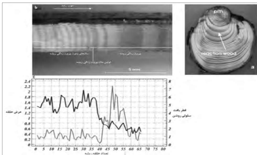
شکل ۲: نمونه دیسک (a) و مغزی (b) از ریشه برونزد یافته و نمودار رشدی آن (c) که نمودار کم‌رنگ عرض حلقه‌های رشدی به میلی‌متر و نمودار پرنگ قطر بافت سلولی روشن در چوب اولیه که برحسب میکرون \times 100 است (کارارا و کارول، ۱۹۷۹: ۳۰۹؛ بادکیو و همکاران، ۲۰۰۵: ۸۷-۹۶).
