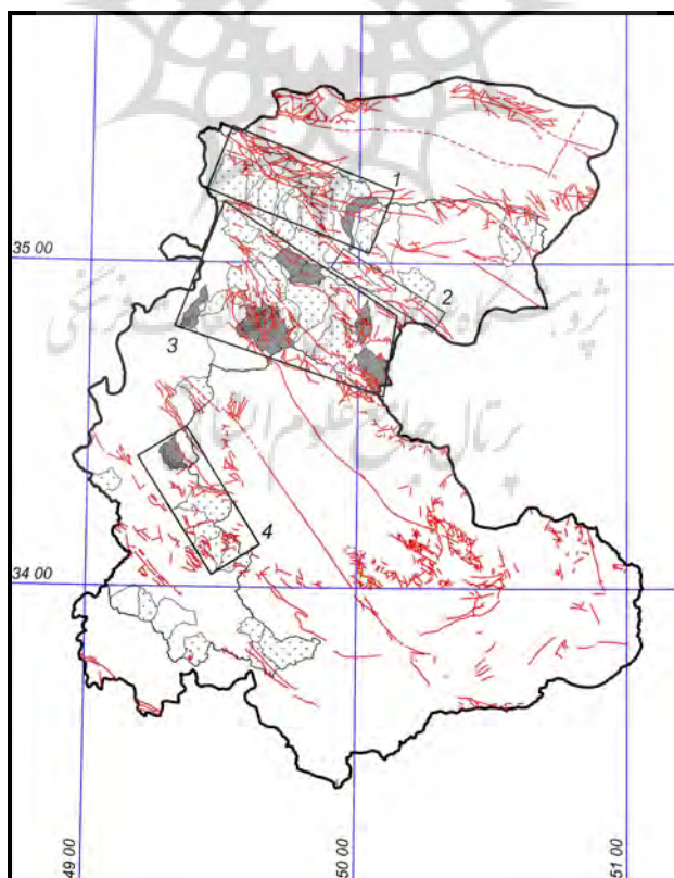
شکل ۹: نقشه وضعیت جنبایی و پراکندگی گسل‌های منطقه
