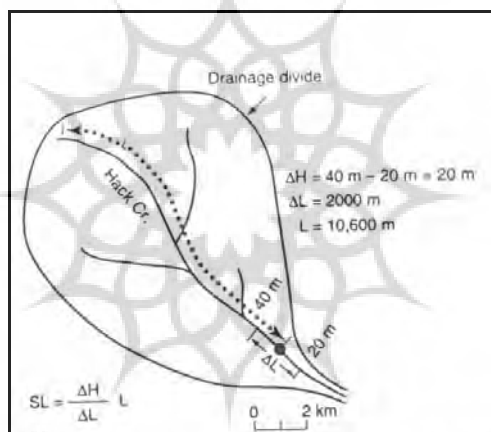
شکل ۲: مواردی که باید در بررسی شاخص آهنگ نشیب رود (SL) اندازه‌گیری شود.
