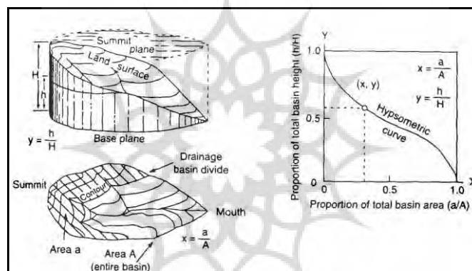
شکل ۳: چگونگی اندازه گیری متغیرهای هیپسومتری
