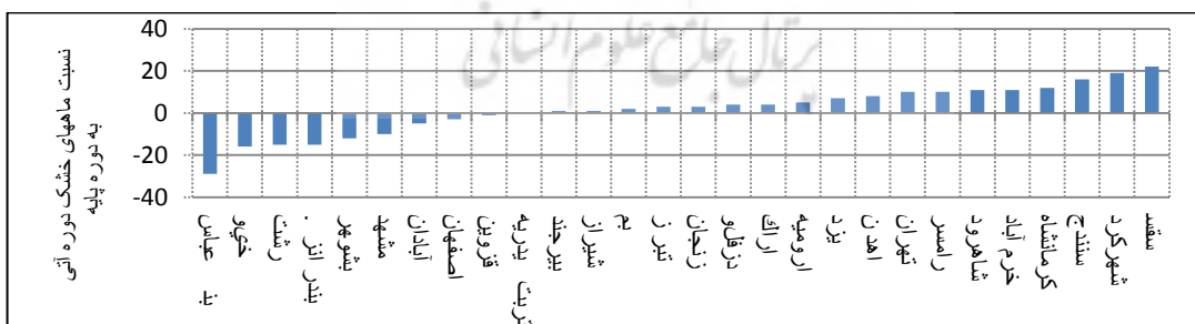
شکل ۲: نسبت فراوانی خشکسالی ایستگاههای منتخب دوره پایه و دوره ۲۰۱۱-۲۰۴۰ براساس مدل Had CM3 و سناریوی A1B برای مقیاس زمانی ۳ ماهه
