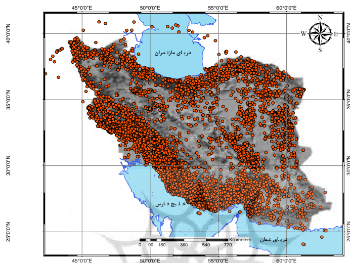
شکل ۳. زلزله‌های ایران با بزرگای بیش از ۴ ریشتر ثبت شده با شبکه‌ی لرزه‌نگاری مؤسسه‌ی ژئوفیزیک دانشگاه تهران که بر روی مدل ارتفاعی رقومی (DEM) کشور قرار گرفته است.
