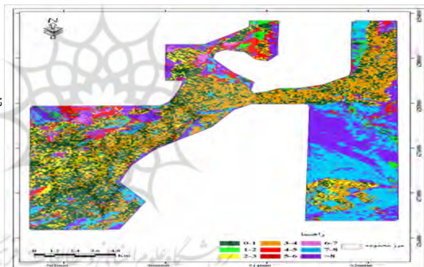
نگاره ۴: پراکنش شوری خاک سطحی به روش طبقه بندی حداکثر احتمال
