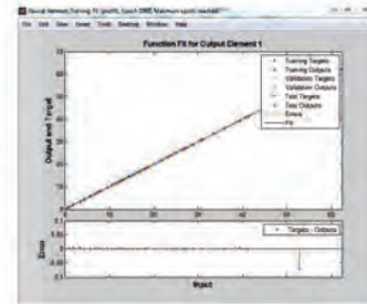
fit
