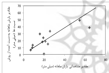
شکل (۵). مقادیر محاسباتی بارش ماهانه به‌دست آمده از روش نسبت‌ها نسبت به مقادیر مشاهداتی
