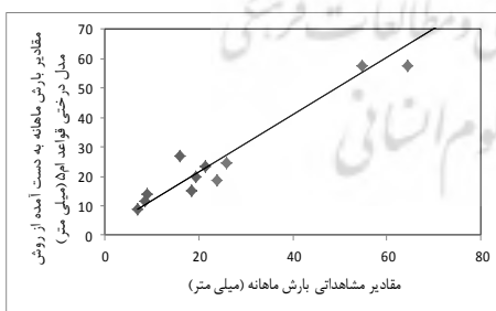
شکل (۷). مقادیر محاسباتی بارش ماهانه به‌دست آمده از روش نسبت‌ها نسبت به مقادیر مشاهداتی
