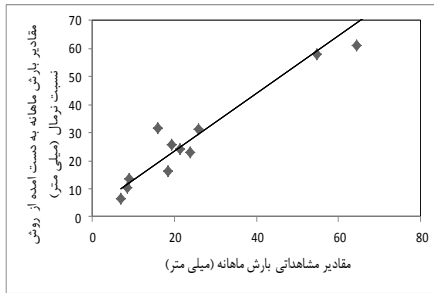
شکل (۳). مقادیر محاسباتی بارش ماهانه به‌دست آمده از روش نسبت نرمال نسبت به مقادیر مشاهداتی
