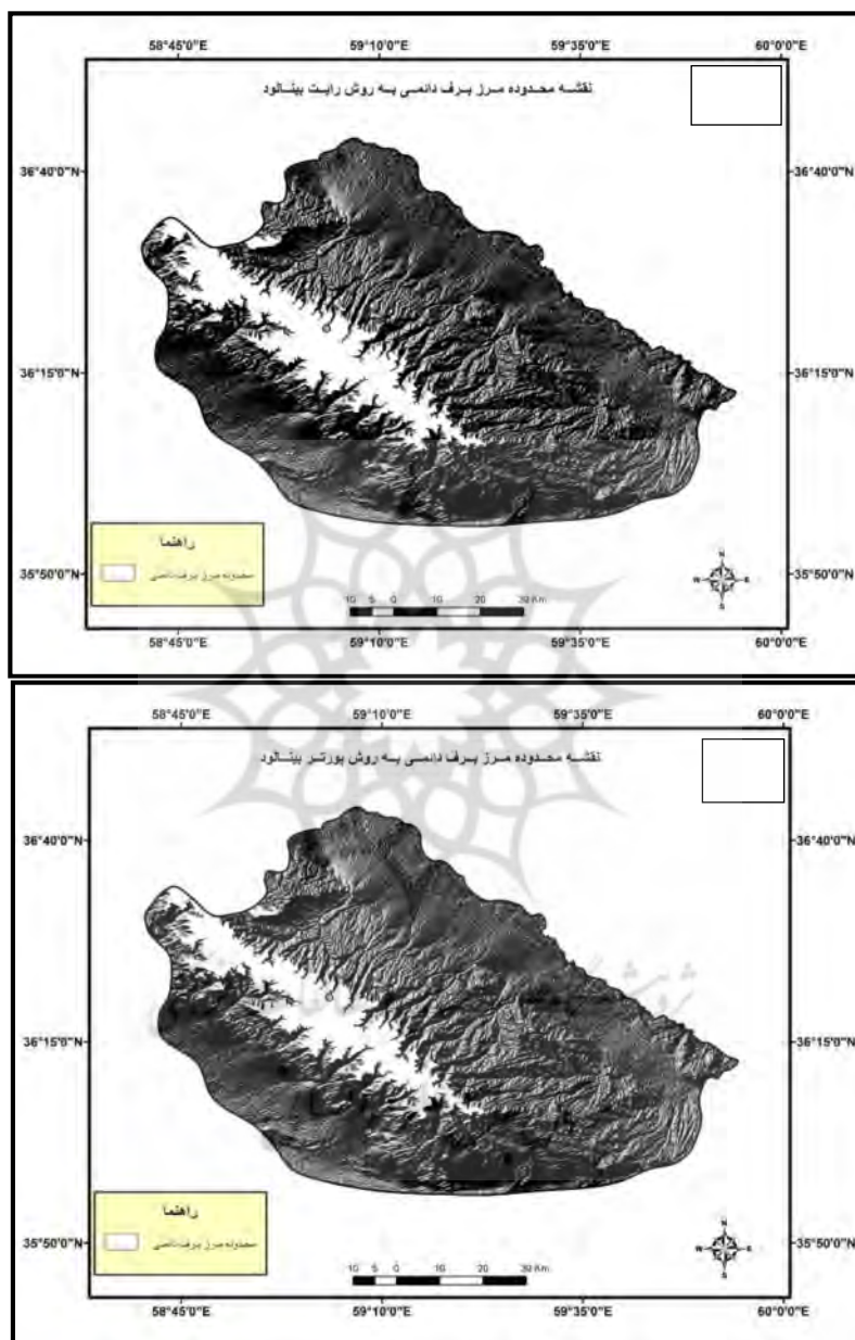
شکل ۸: الف: نقشه محدوده برف‌مرز به روش رایت ب: نقشه محدوده برف‌مرز به روش پورتز
