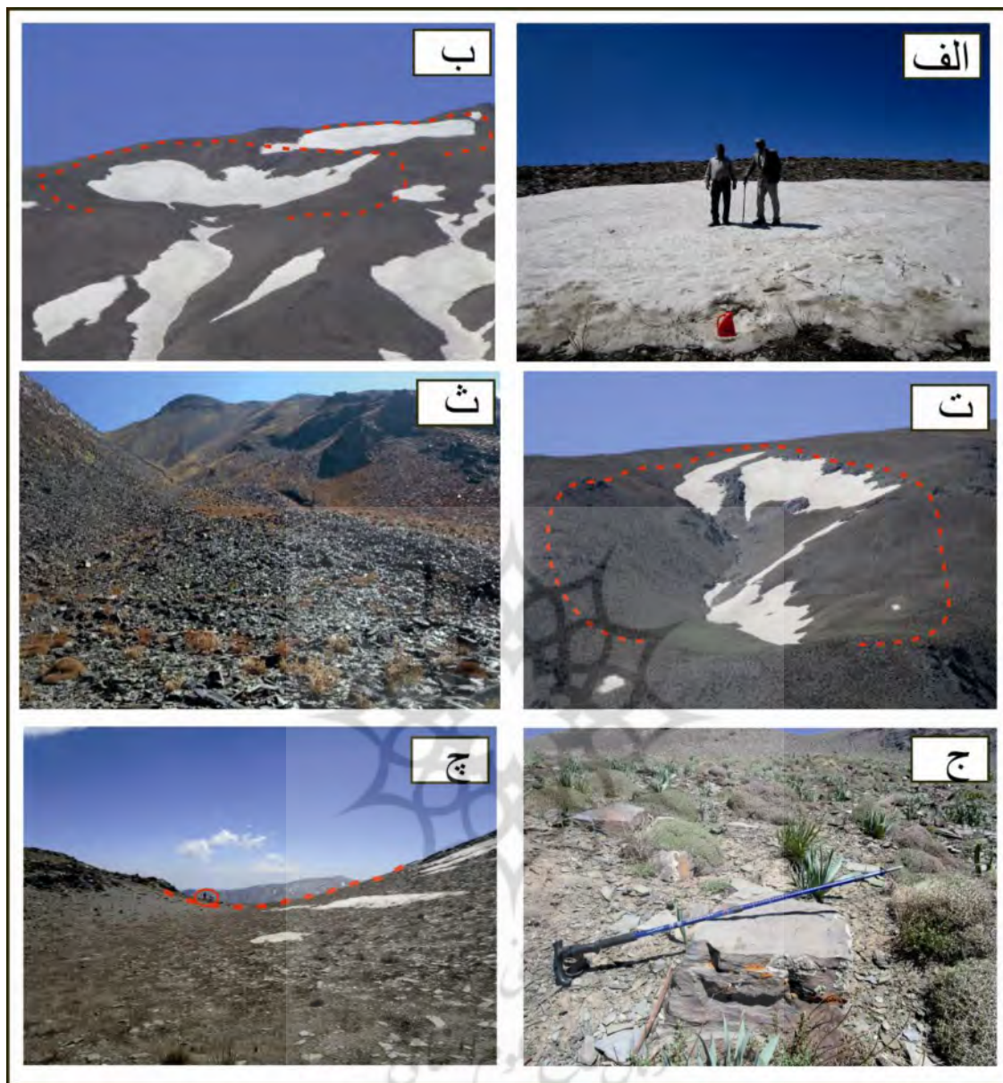
شکل ۳: الف) (ب و ت) - سیرک‌های یخچالی و آثار باقی‌مانده. ث) - تیل یا یخرفت در ارتفاعات محدوده مورد مطالعه ج). تخته‌سنگ‌های بجا مانده از فعالیت‌های یخچالی در محدوده مورد مطالعه. ج) - آثار دره‌های یخچالی گسترش نیافته
