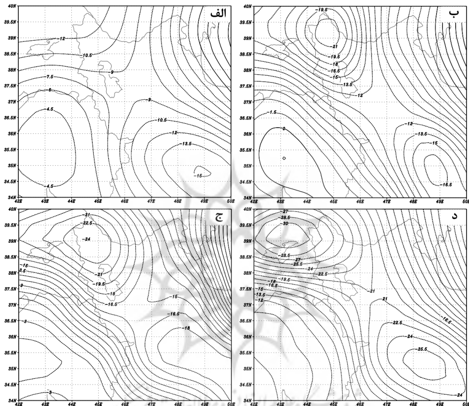
شکل (۶). حداقل دمای ۲ متری سطح زمین برای (الف) روز ۱۲ دسامبر ۱۹۶۳ (طبقه امواج سرد ضعیف)، (ب) روز ۱۱ ژانویه ۱۹۸۳ (طبقه امواج سرد متوسط)، (ج) روز ۷ ژانویه ۱۹۸۹ (طبقه امواج سرد بسیار شدید)، (د) روز ۲۰ ژانویه ۱۹۶۴ (طبقه امواج ابر سرد). در شکل دما به درجه سانتی گراد بیان شده است.
