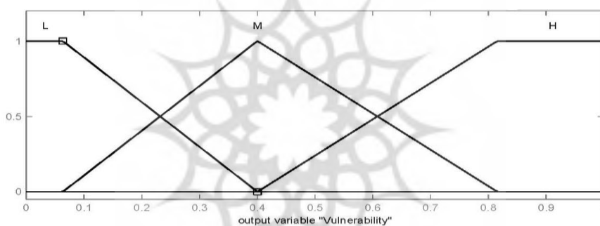
شکل ۴. توابع عضویت خروجی نهایی (میزان آسیب‌پذیری)
