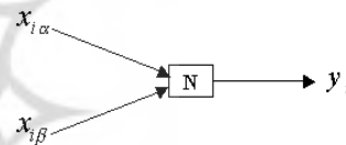
شکل ۲- ساختار نرون
