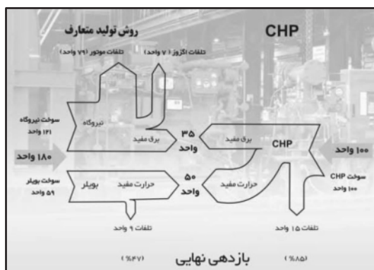
شکل ۵- مقایسه شماتیک تولید برق به روش متعارف و نیروگاه مقیاس کوچک گازی
