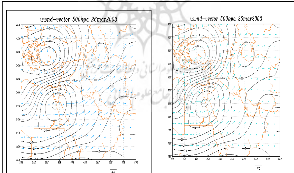
شکل ۳- نقشه بردار باد و خطوط هم سرعت تراز ۵۰۰ هکتوپاسکال مربوط به روزه های گردوغباری
