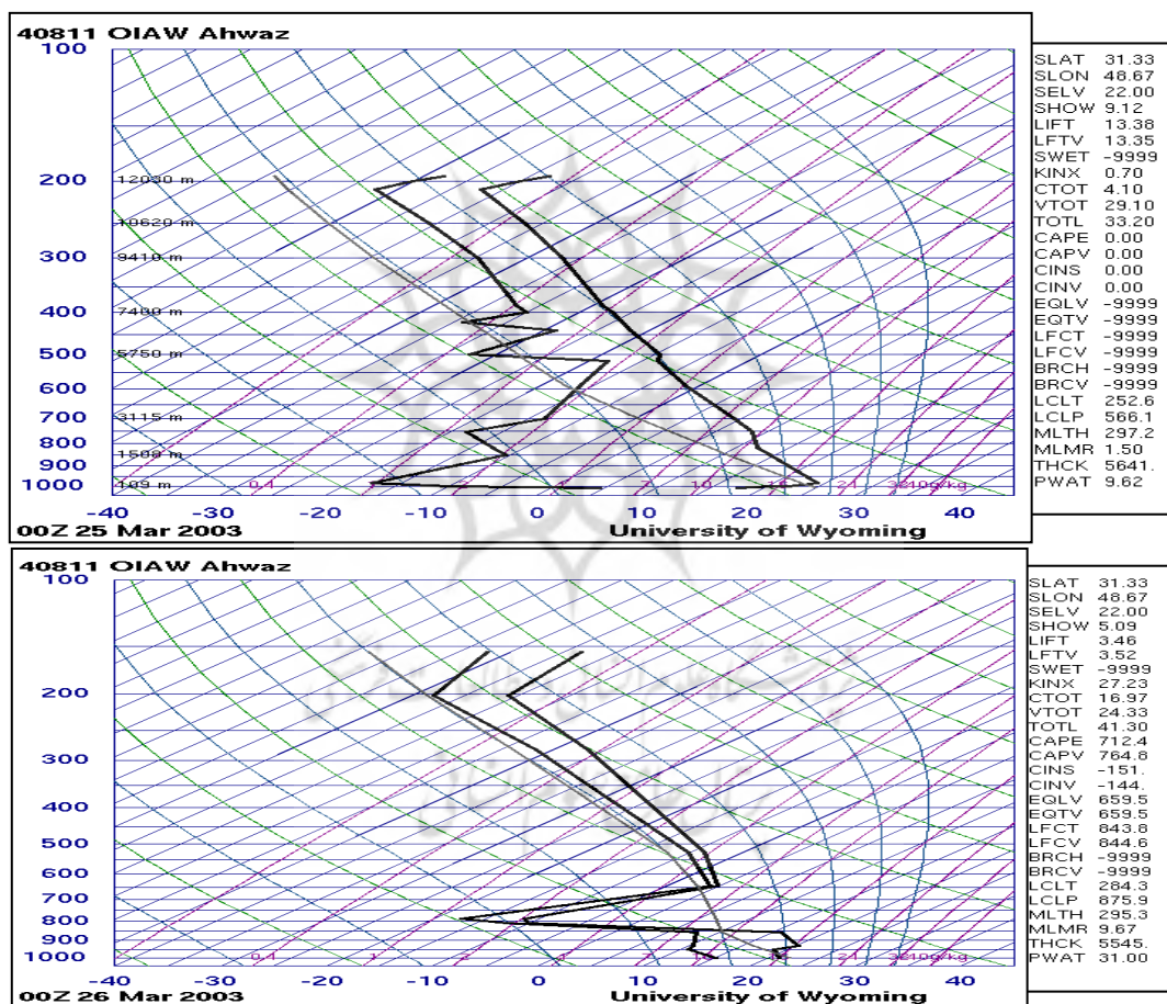
شکل ۹- نمودار اسکیتوی ایستگاه جوبالا اهواز در روز ۲۵ مارس ۲۰۰۳ برای ساعت ooutc ، روز قبل از توفان ۲۶ مارس ۲۰۰۳ برای ساعت ooutc ، روز اوج توفان
