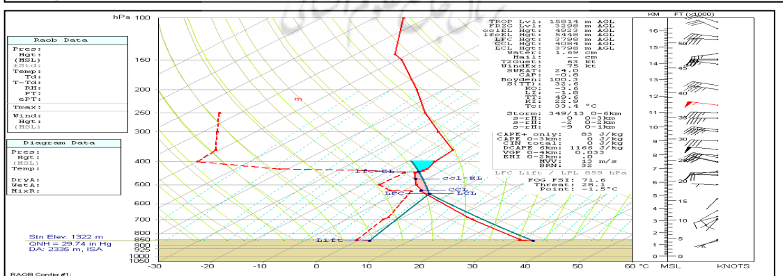
شکل ۱۳- نمودار اسکایوتی ایستگاه جو بالا کرمانشاه در روز ۳۰ ژوئن ۲۰۰۸ ساعت ۰۰ UTC و ۱۲ UTC و ۱ جولای ۲۰۰۸ ساعت ۰۰ UTC (با استفاده از نرم افزار RAOB)
