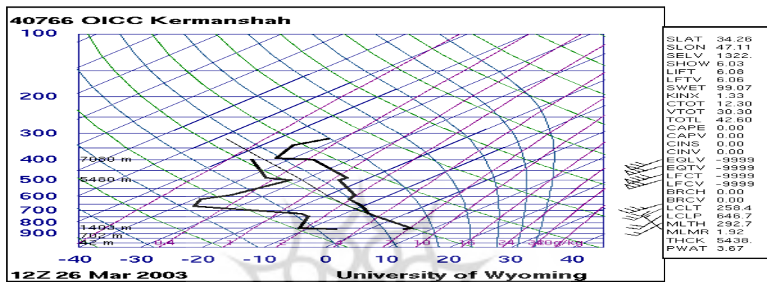
شکل ۱۰- نمودار های اسکیتوی ایستگاه جوپالا کرمانشاه در روز ۲۵ مارس ۲۰۰۳ برای ساعت 12ute، روز قبل از توفان و در روز ۲۶ مارس ۲۰۰۳ برای ساعت 12ute، روز اوج توفان
