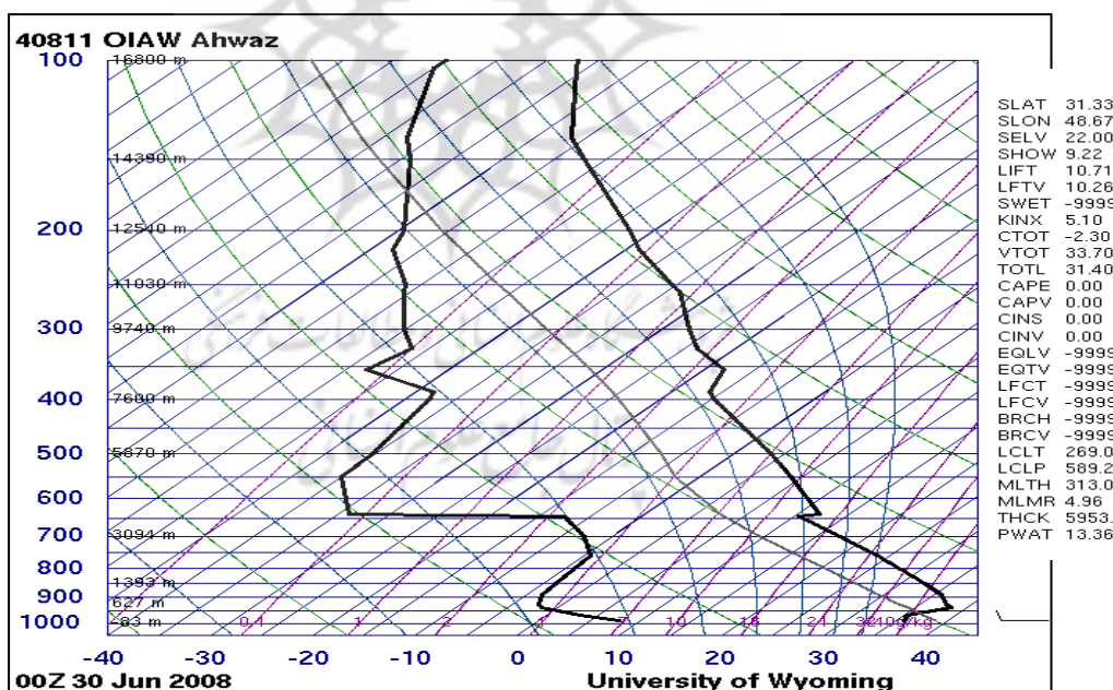
شکل ۱۲- نمودار اسکیتوی ایستگاه جو بالا اهواز در روز ۳۰ ژوئن ۲۰۰۸ ساعت 00UTC
