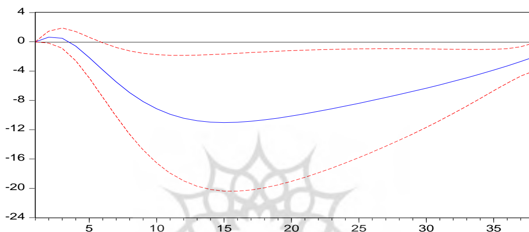
شکل (۱) نمودار نتایج تابع واکنش آنی شاخص قیمت بازار سهام به قیمت نفت
