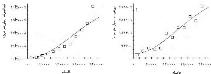
شکل ۴. نیم تغییرنمای تجربی (مربع توخالی) و بهترین الگوی برازش شده (خط ممتد) مربوط به متغیرهای کمکی ارتفاع (الف) و فاصله تا خط ساحلی (ب)
