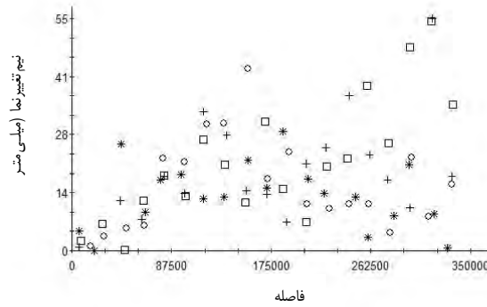
شکل ۲. نیم تغییرنمای جهت‌دار بارندگی خرداد
