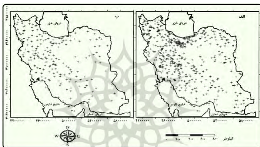
شکل ۱: پراکنش ایستگاه‌های به‌کار رفته در تهیه‌ی پایگاه داده‌ی اسفزاری (الف) و تکمیل آن (ب)
