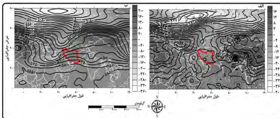
شکل ۸: توزیع مکانی فشار تراز دریا به هکتوپاسکال (الف) و توزیع مکانی ارتفاع تراز ۵۰۰ هکتوپاسکال به متر (ب)
