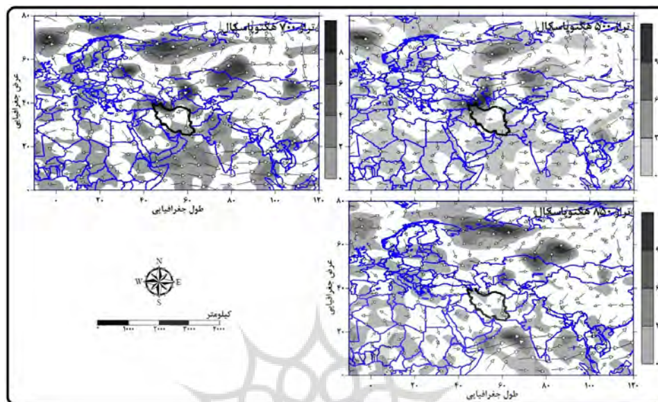
شکل ۵: وزش دمایی روز نماینده گروه اول در ترازهای مختلف جو به گرم در مترمکعب در روز
