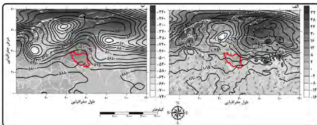
شکل ۱۰: توزیع مکانی فشار تراز دریا به هکتوپاسکال (الف) و توزیع مکانی ارتفاع تراز ۵۰۰ هکتوپاسکال به متر (ب)
