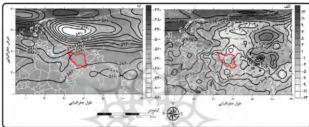
شکل ۴: توزیع مکانی فشار تراز دریا به هکتوپاسکال (الف) و توزیع مکانی ارتفاع تراز ۵۰۰ هکتوپاسکال به متر (ب)
