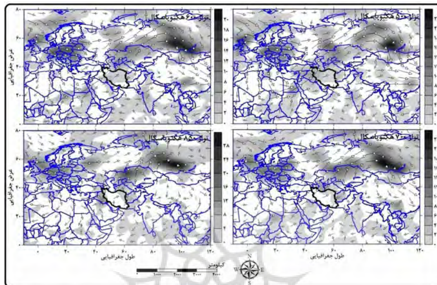
شکل ۷: وزش دمایی روز نماینده گروه دوم در ترازهای مختلف جو به گرم در مترمکعب در روز
