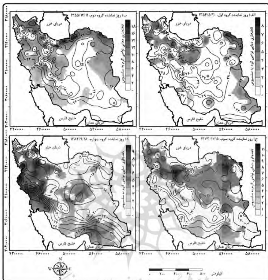
شکل ۳: توزیع مکانی میانگین دمای روزهای گرم (همدمها) و ناهنجاری آن (پس‌زمینه) برای روزهای نماینده
