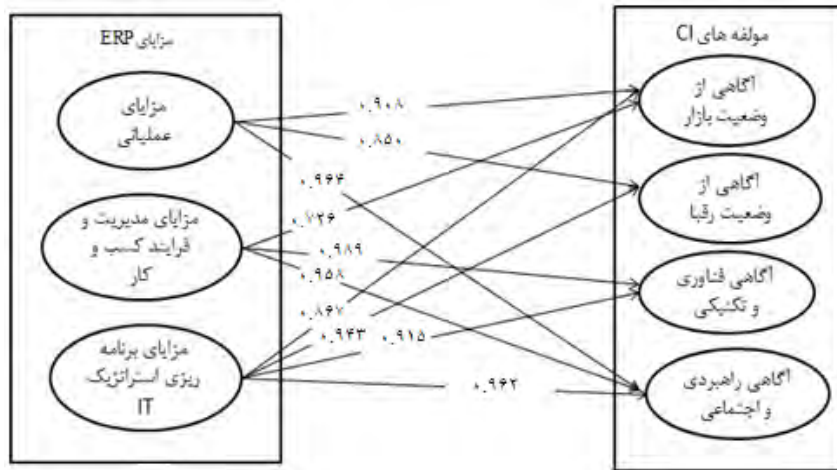
شکل ۳. نتایج فرضیه‌ها
