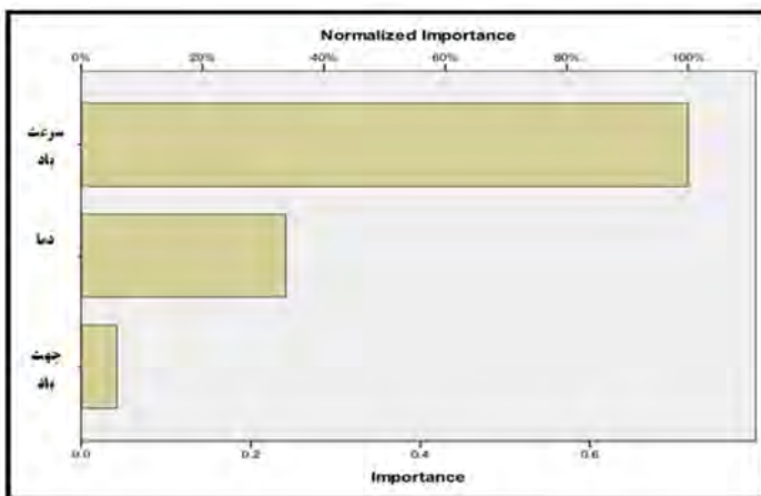
نگاره ۵: اهمیت پارامترهای هواشناسی مورد استفاده در تخمین آلودگی هوا در شبکه عصبی پژوهش
