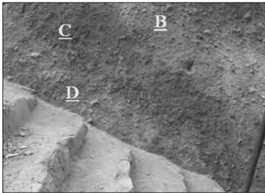
تصاویر ۸ و ۹: برخی گونه‌های شاخص آسیب سنگ در معماری صخره‌ای کندوان. (A) تورق شدید با بیش از ۵ سانتی‌متر جدایش از بستر اصلی. (B) از دست رفتن زمینه (C) تغییر رنگ و تاول (D) جدایش دانه‌ای (مأخذ: نگارندگان ۱۳۹۲).
