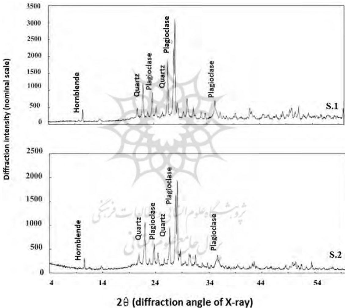
نمودار ۱: نمودارهای آنالیز (XRD) سنگ سالم ایگنیمبریت خانه‌های صخره‌ای روستای کندوان
