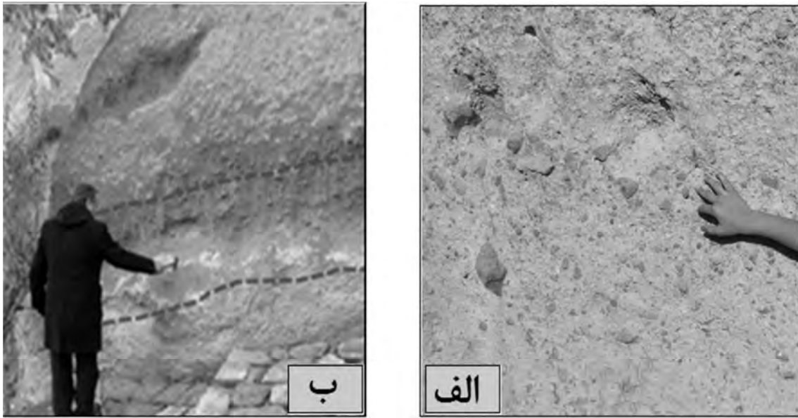
تصویر ۵: توده سنگ و (ب) میان لایه‌های فرسایش یافته در توده سنگ روستای کندوان (مأخذ: نگارندگان ۱۳۹۲)
