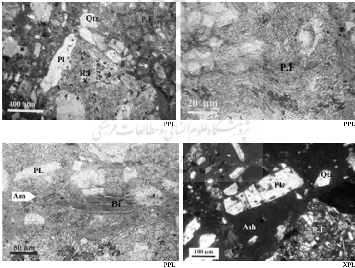
تصویر ۶: تصاویر مقاطع میکروسکوپی از سنگ کندوان (مأخذ: نگارندگان) P.F: قطعات پامیس؛ R.F: قطعات سنگی؛ Qtz: کوارتز؛ PL: آنورتیت (پلاژیوکلاز)؛ Bi: بیوتیت؛ Am: هورنبلند (آمفیبول)
