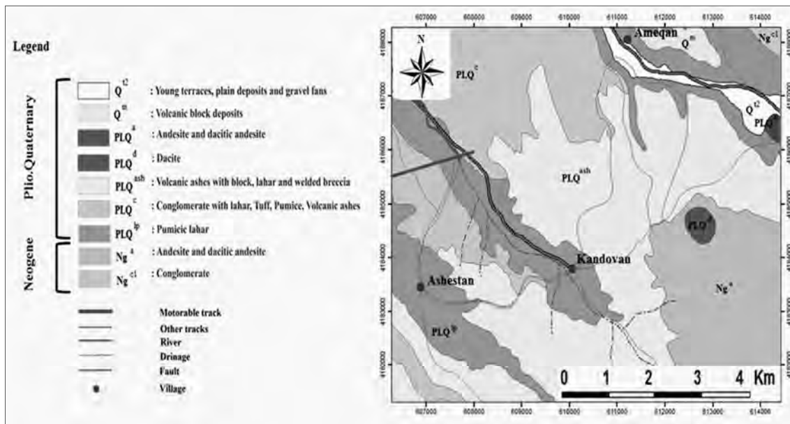
تصویر ۲: موقعیت روستای کندوان در دامنه کوه سه‌هند در بستر زمین‌شناسی منطقه (مأخذ: خدابنده و امینی فضل، ۱۳۷۴).
