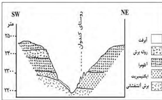
تصویر ۳: الف) تصویر هوایی از دره و روستای کندوان. ب) محل قرارگیری روستا در میان لایه‌های مقطع زمین‌شناسی دره کندوان. (مأخذ تصویر: Google Earth, 2013; مأخذ مقطع دره: معین وزیری، ۱۳۷۷: ۱۲۶)
