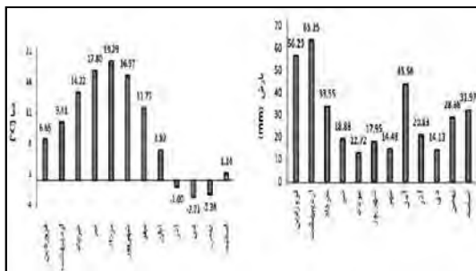
تصویر ۴: نمودار میزان بارش و درجه حرارت متوسط ماهانه برای دوره ده ساله (۱۳۷۹ - ۱۳۸۸) (مأخذ: امینی بیرامی، ۱۳۹۲)
