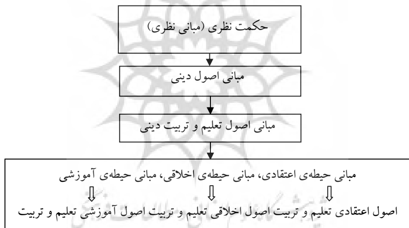
شکل ۵. مدل مفهومی
