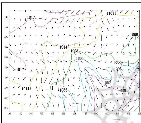
شکل ۵. نقشه‌ی فشار سطح دریا (هکتوپاسکال) و بردار باد (متر بر ثانیه) منطقه‌ی خاورمیانه (۱۰ تیرماه ۱۳۸۸)
