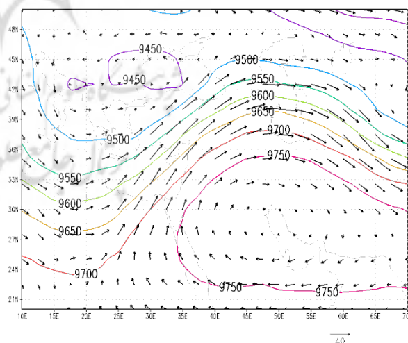
شکل ۹. نقشه ی ارتفاع ژئوپتانسیل (متر) و بردار باد (متر بر ثانیه) سطح ۳۰۰ هکتوپاسکال منطقه ی خاورميانه (۹ تيرماه ۱۳۸۸)
