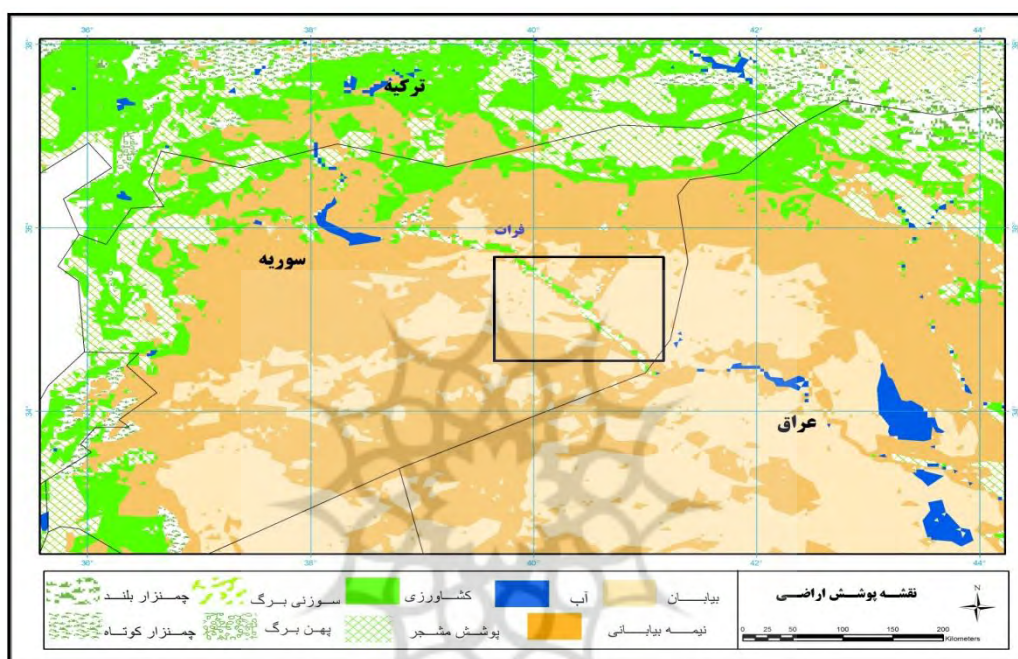
شكل ۳. نقشه‌ي پوشش سطح زمين ناحیه‌ي تشكيل توفان از داده‌هاي مورد استفاده در مدل RegCM
