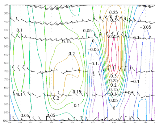
شکل ۱۰. نیم‌رخ قائم (سطح ۱۰۰۰ تا ۳۰۰ هکتوپاسکال) باد (متر بر ثانیه) و مقادیر اُمگا (ω) برای عرض ۳۵ درجه‌ی شمالی در منطقه‌ی خاورمیانه (۹ تیرماه ۱۳۸۸)
