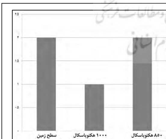
شکل ۷. میزان تغییر سرعت باد (متر بر ثانیه) روز ۱۰ تیرماه نسبت به روز پیش در سطح زمین، ۱۰۰۰ و ۸۵۰ هکتوپاسکال در منطقه‌ی تشکیل توفان
