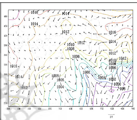
شکل ۴. نقشه‌ی فشار سطح دریا (هکتوپاسکال) و بردار باد (متر بر ثانیه) منطقه‌ی خاورمیانه (۹ تیرماه ۱۳۸۸)
