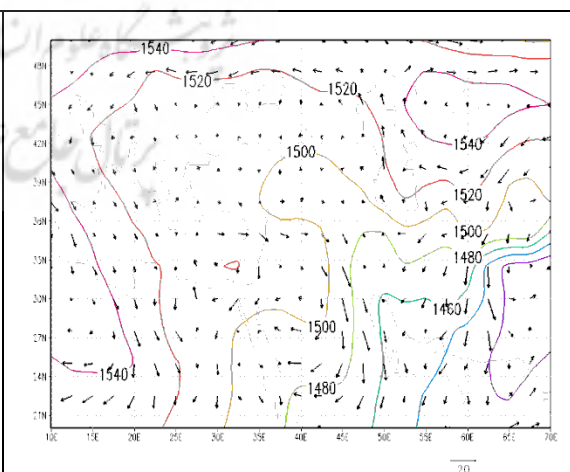
شکل ۶. نقشه‌ی ارتفاع ژئوپتانسیل (متر) و بردار باد (متر بر ثانیه) سطح ۸۵۰ هکتوپاسکال منطقه‌ی خاورمیانه (۹ تیرماه ۱۳۸۸)
