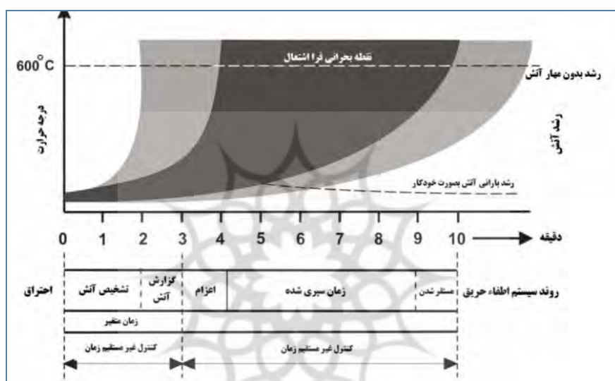
شکل ۱. روند سیستم اطفای حریق به همراه زمان رسیدن به نقطه فراشتعالی
