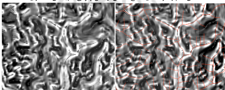
شکل ۹- پارامتر انحنای مقطع حاصل از مدل رقومی
