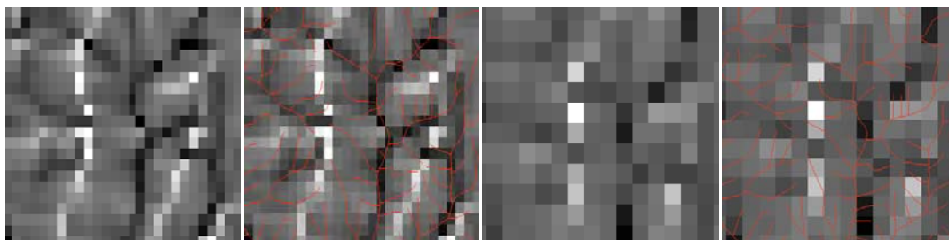
شکل ۶- پارامتر انحنای سطح حاصل از مدل رقومی شکل
