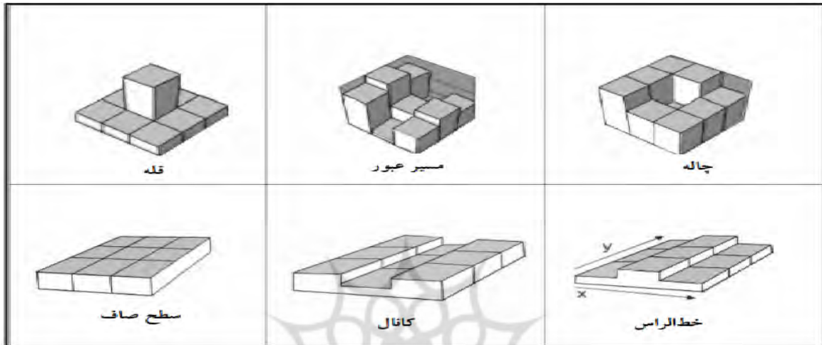
شکل ۲- شش نوع ویژگی مورفومتری
