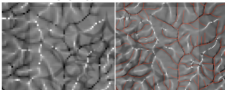
شکل ۸- پارامتر انحنای سطح حاصل از مدل رقومی با پیکسل ۱۰ متری
