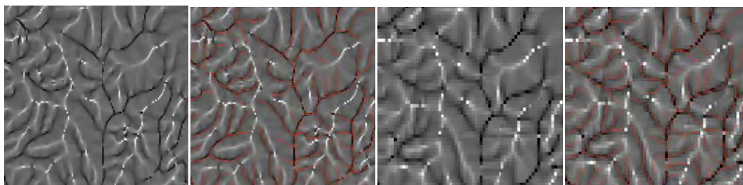
شکل ۴- پارامتر انحنا (Plan Curvature) سطح حاصل از مدل رقومی با پیکسل ۱۰ متری
