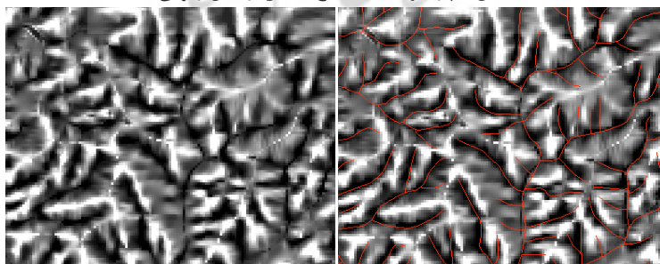
شکل ۱۰- پارامتر انحنای متقاطع حاصل از مدل رقومی با پیکسل ۱۰ متری
