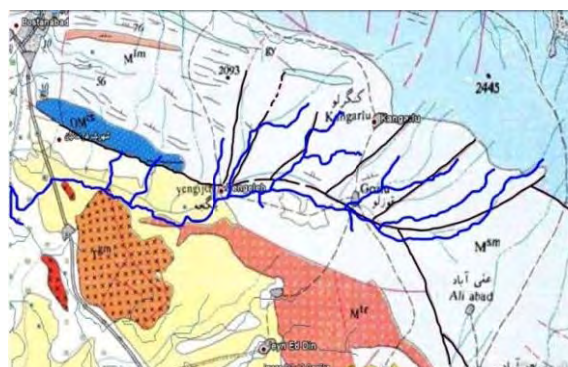
شکل ۸. زیر حوضه شماره ۶ را نشان می‌دهد. در این شکل قطع‌شدگی شبکه زهکشی توسط خطوط گسلی به خوبی نشان داده شده است. تحت تاثیر شبکه گسلی بخش سمت راست حوضه بالا آمادگی داشته و شبکه آبراهه یک جابجایی به سمت چپ حوضه داشته است.
