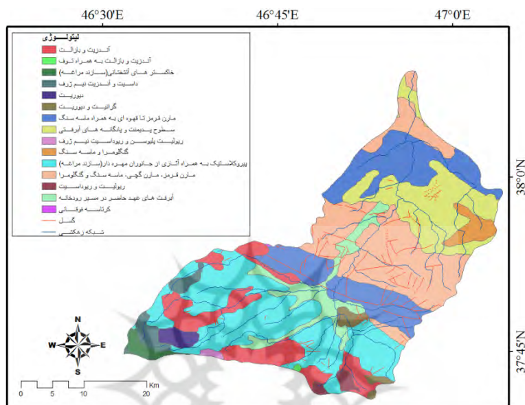
شکل ۲. نقشه زمین‌شناسی حوضه آبریز اوجان چای
