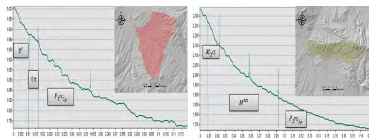
شکل ۱۳. نیمرخ طولی زیر حوضه ۵
