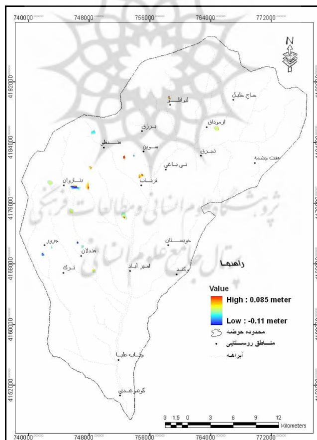
شکل ۳: نقشه مناطق ناپایدار و میزان جابجایی آن‌ها در حوضه گرم چای به روش اینترفرومتری تفاضلی زوج تصویر
