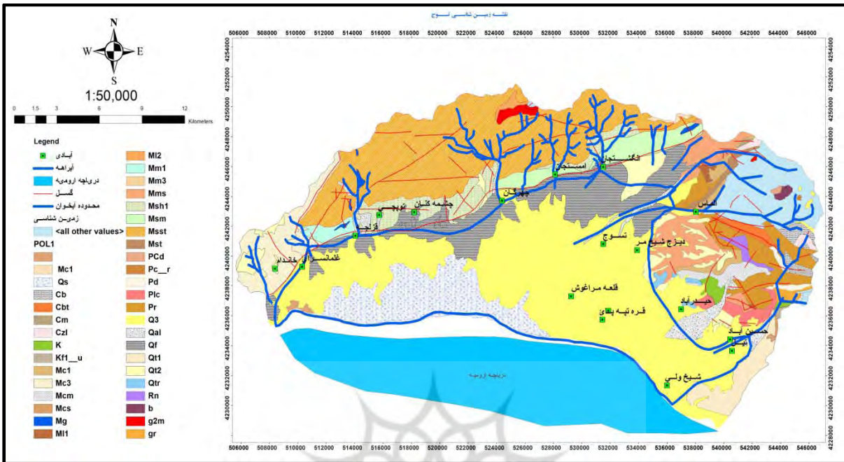
شکل ۳ - نقشه زمین‌شناسی محدوده مطالعاتی (اقتباس از نقشه زمین‌شناسی ۱/۱۰۰۰۰۰ تسوج)
