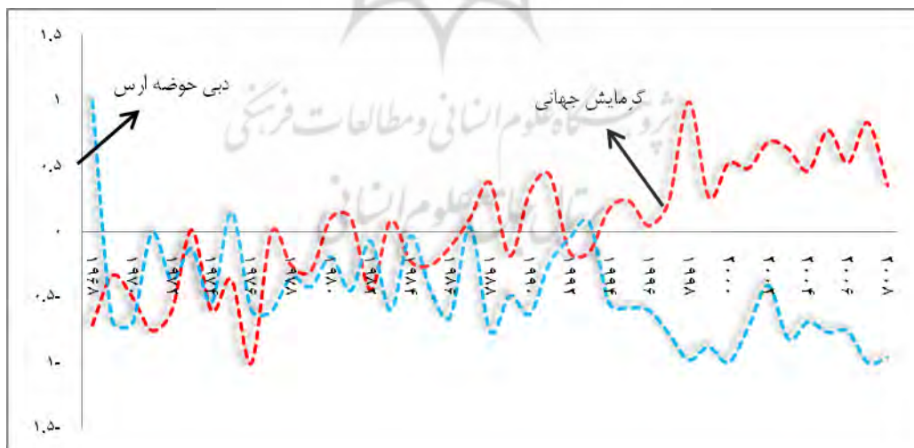
شکل ۱۰. نمودار استاندارد شده نوسان‌های بلند مدت فصل بهار دبی حوضه آرس و گرمایش جهانی طی بازه زمانی چهار ساله
