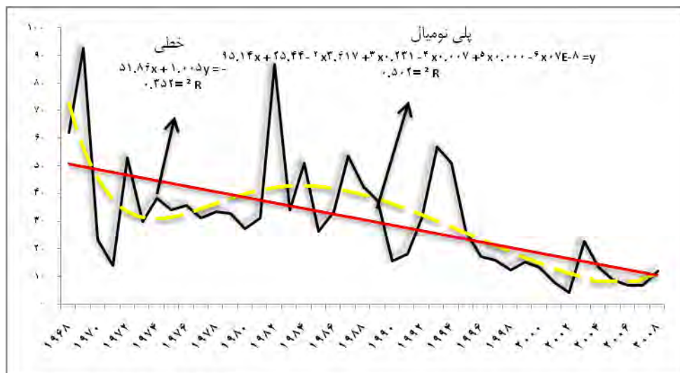
شکل ۱۷. تغییرات سری زمانی فصل پاییز دبی حوضه ارس طی بازه زمانی چهل ساله
