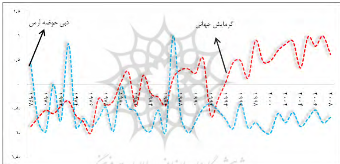
شکل ۱۳. نمودار استاندارد شده نوسان‌های بلندمدت فصل تابستان دبی حوضه ارس و گرمایش جهانی طی بازه زمانی چهل‌ساله
