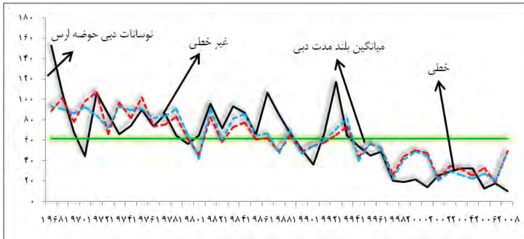
شکل ۹. نمودار برآورد شده رگرسیون خطی و غیرخطی با میانگین بلندمدت و نوسان‌های دبی حوضه آرس در فصل بهار
