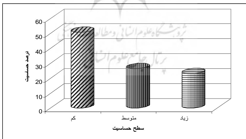
شکل ۹. نمودار توزیع سطوح مختلف حساسیت به کارست بر اساس درصد مساحت در منطقه‌ی شاهو
