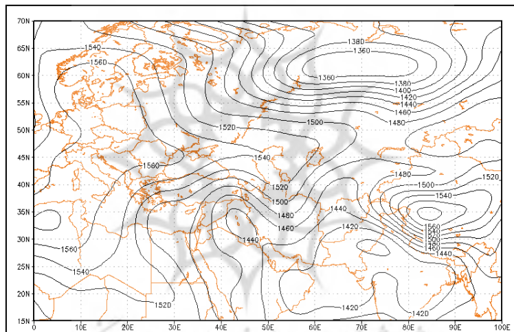
شکل ۵ الگوی آرایش متوسط توپوگرافی ارتفاع ژئوپتانسیل ترازهای ۸۵۰ هکتوپاسکال از ۹ تا ۱۵ مرداد ۱۳۸۷
