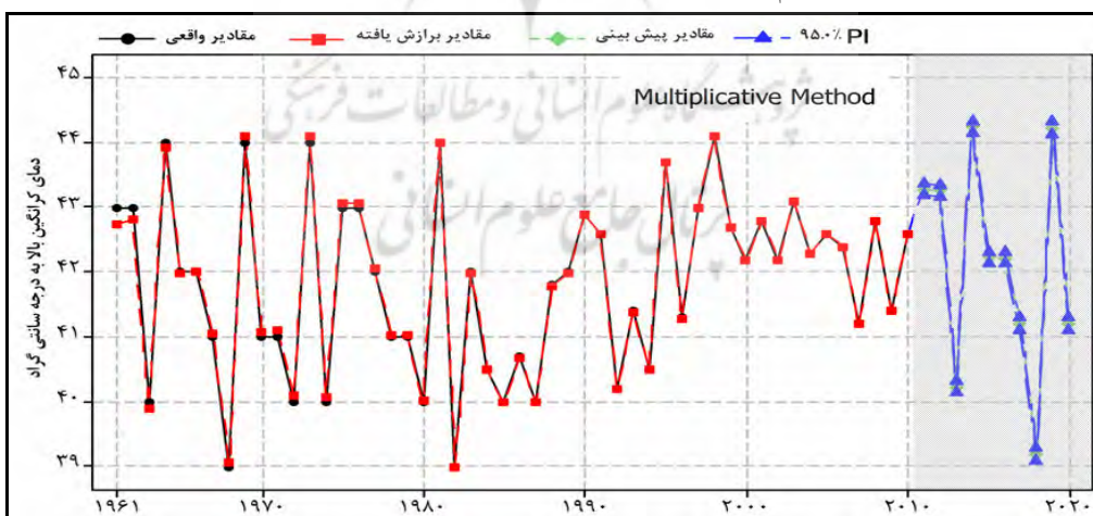
شکل ۸ پیش‌بینی دماهای کرانگین بیشینه تا سال ۲۰۲۰ با استفاده از مدل حالت-ویترز
