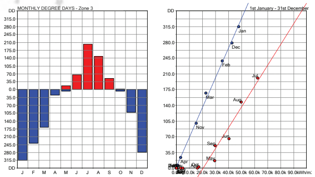
نمودار (۳) محاسبه درجه روز در ماه‌های مختلف سال برای بخش سه ساختمان نمونه طراحی شده در تهران
