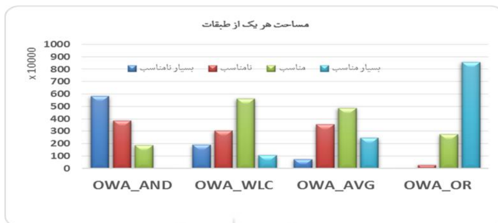
شکل ۴) نمودار ستونی مقادیر OWA جهت شناسایی مکان‌های مناسب توریین‌های بادی
