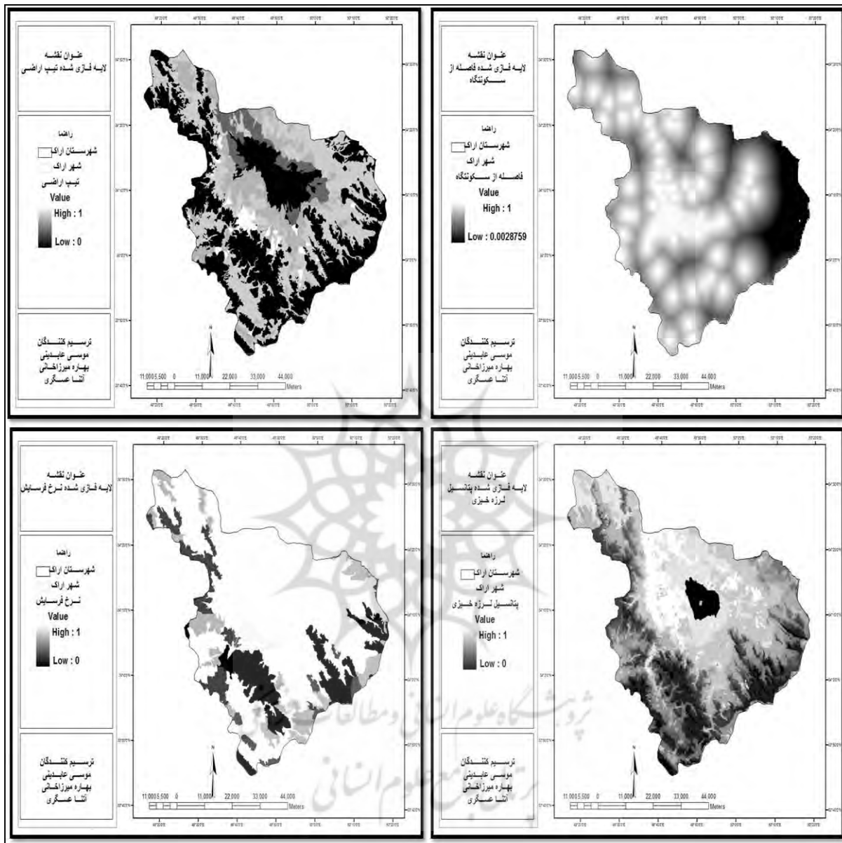
شکل ۳- لایه های فازی شده براساس توابع فازی: ۱- فاصله از سکونتگاه ۲- میزان فرسایش پذیری ۳- پتانسیل لرزه خیزی
