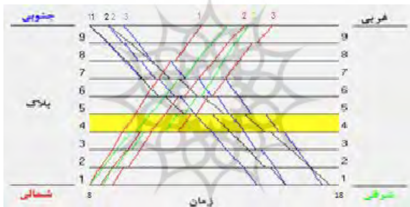
شکل ۲) - نمودار حرکت قطار در دو مسیر متقاطع
