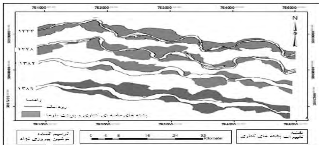
شکل (۱۲) تغییر مساحت پشته کناری از مئاندری به گیسویی در بازه ۴ رودخانه گاماسیاب
