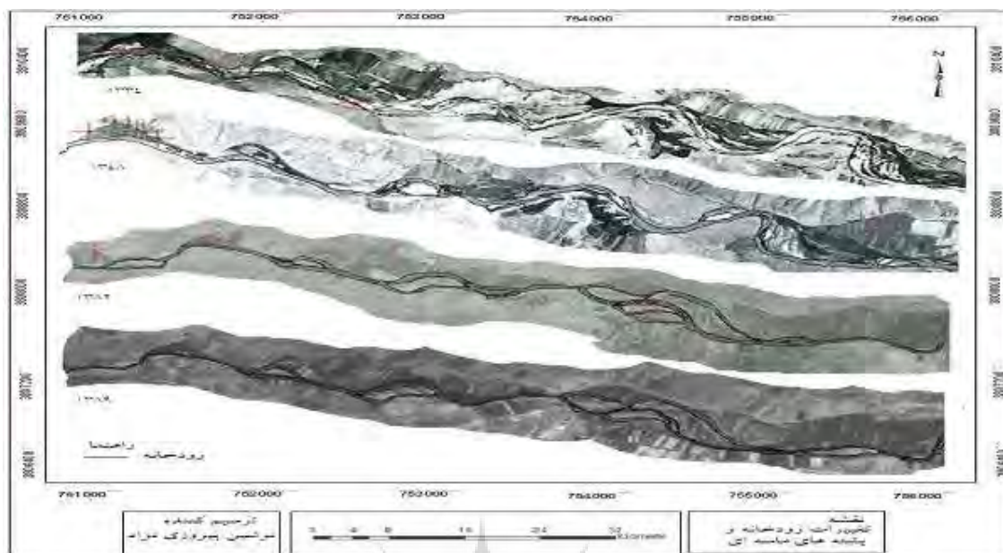
شکل (۳) روند تغییرات الگوی رودخانه و مساحت پشته‌های ماسه ای در بازه ۱ و ۲
