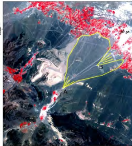
شکل ۲) جابه‌جایی مراکز بیشینه رسوبی روی مخروطه افکنه موغار
