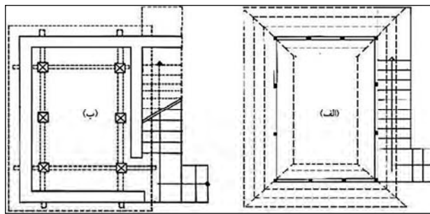
پلان شماره ۲: پلان طبقه فوقانی (الف) و همکف (ب) سقائفار
