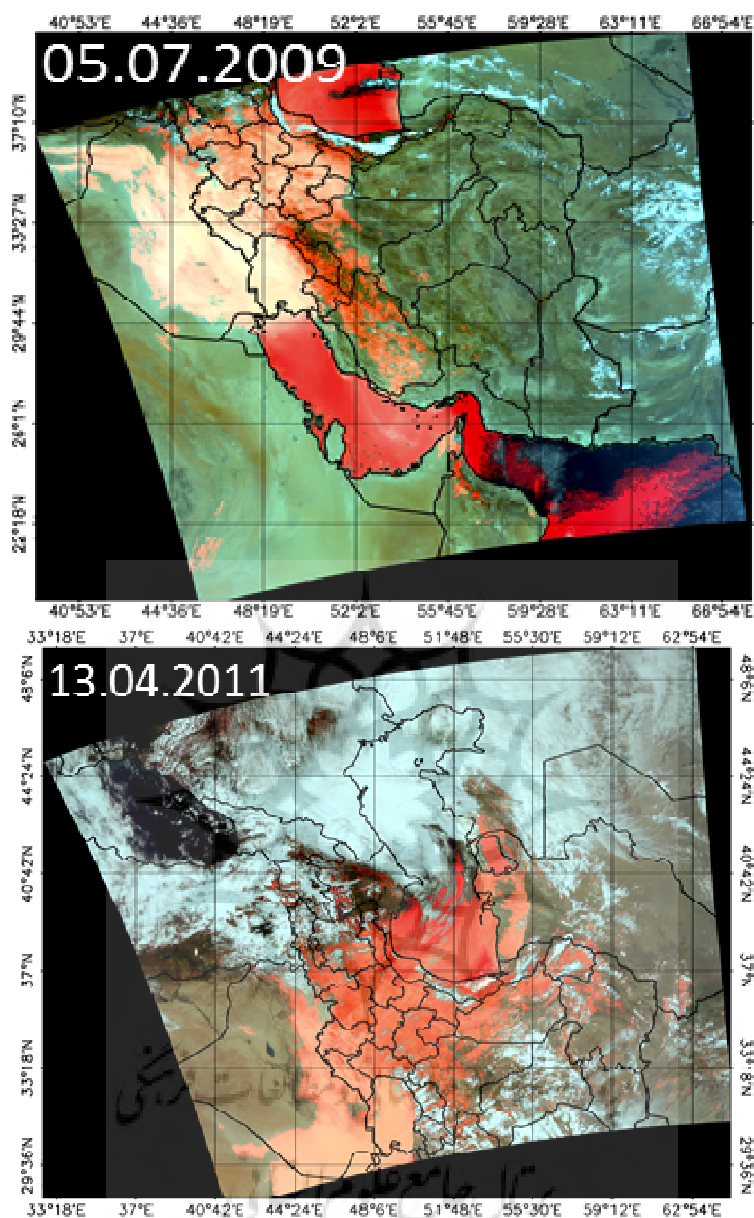
شکل (۵): تصاویر سنجنده مادیس ماهواره‌های تورا و آکوا رخدادهای گرد و غبار در نیمه غربی ایران را نشان می‌دهند. بارزسازی گرد و غبار از طریق ویژگیهای دمای درخشایی و با استفاده از روابط (MNDVI) < 0 and (b31-b32) < 0 (الف: دوره گرم ب: دوره سرد)
