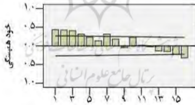
نمودار تابع ACF سری بیرجند
