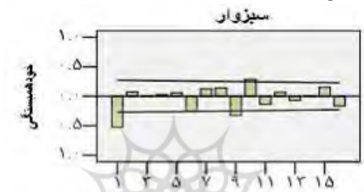
شکل (۱۳) نمودار ACF با تفاضل ۱ سبزووار
