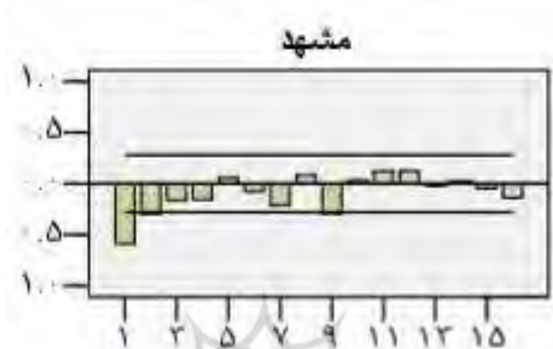
شکل (۴) نمودار خودهمبستگی جزئی سری مشهد
