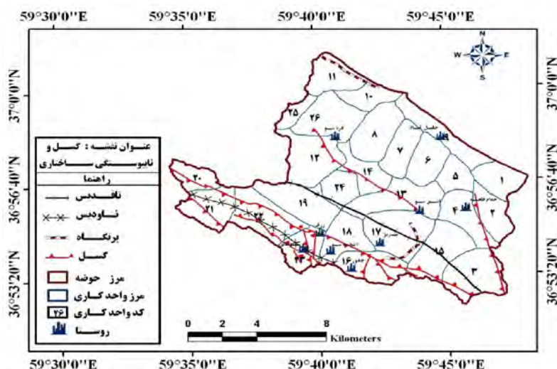
شکل (۷) نقشه گسله و ناپیوستگی ساختاری حوضه آبخیز کلات
