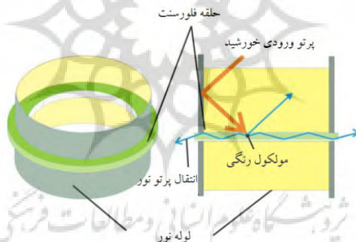
شکل ۱۷ - طرح حلقه های فلورسنت برای استخراج نور [۱]
