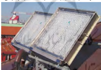
شکل ۸- جمع‌کننده نور خورشید برای سیستم فیبر نوری [۱]
