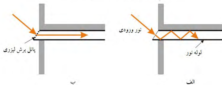
شکل ۱۳: لوله‌های نور افقی
