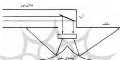
شکل ۲۱ - پخش کننده نور [۱]
