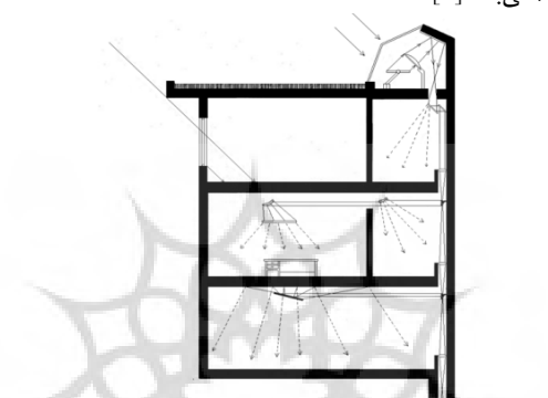
شکل ۱۱ - آرایش عدسی‌ها و آینه‌ها برای انتقال نور روز [۱]
