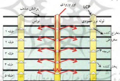
شکل ۱۵ - طرح لوله نور عمودی [۱]
