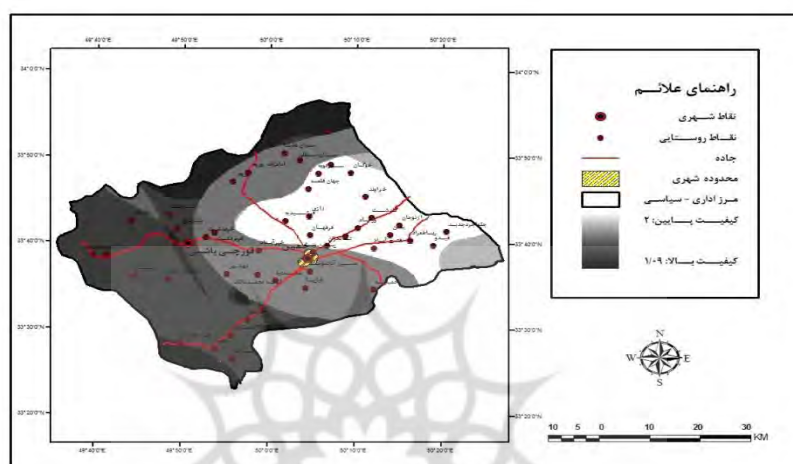
شکل ۴. نقشه رس تری معیار اقلیم
